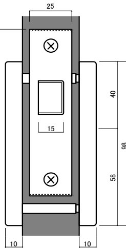
切り欠き図
