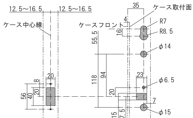
切り欠き図
