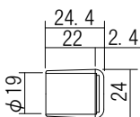
キャップ
