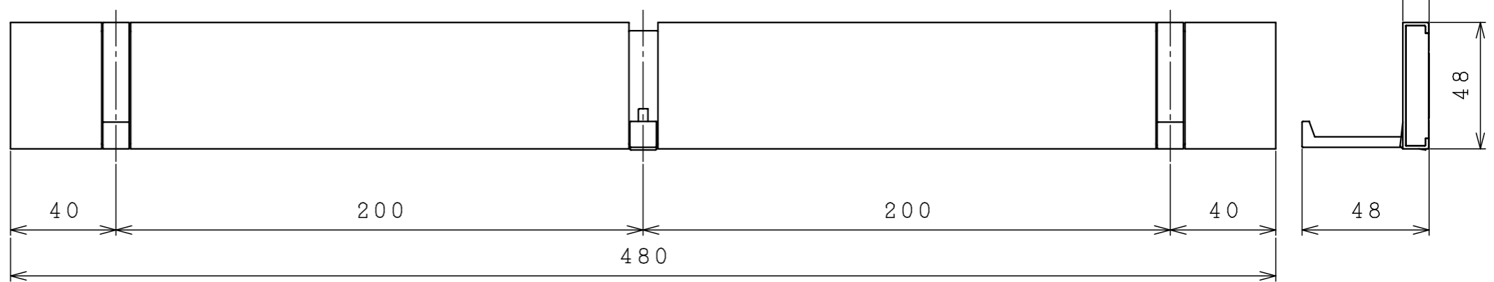
3連フック
