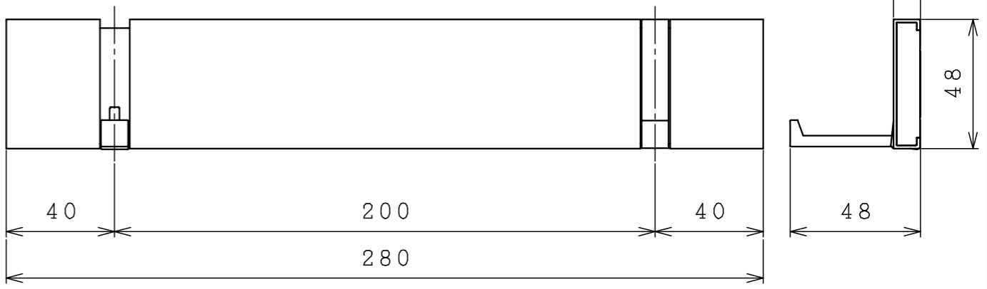
2連フック
