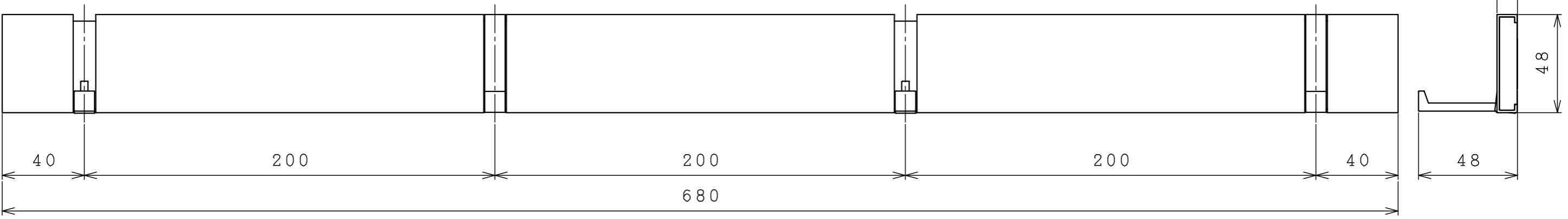
4連フック
